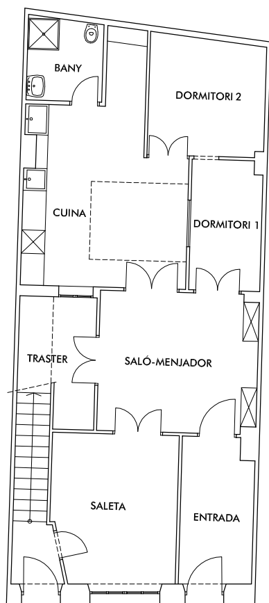
PLANTA BAIXA
